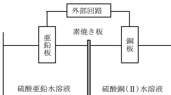
図 ダニエル電池の模式図
